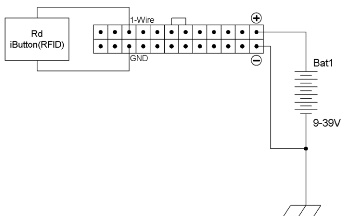
Рисунок 6. Схема подключения считывателей iButton(RFID) для терминалов v5
